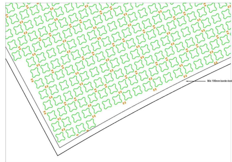
Detalle 2 Escala 1:25
